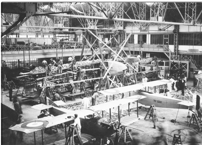
Avions Caudron C-59 en cours de montage dans une usine Caudron vers 1918.
